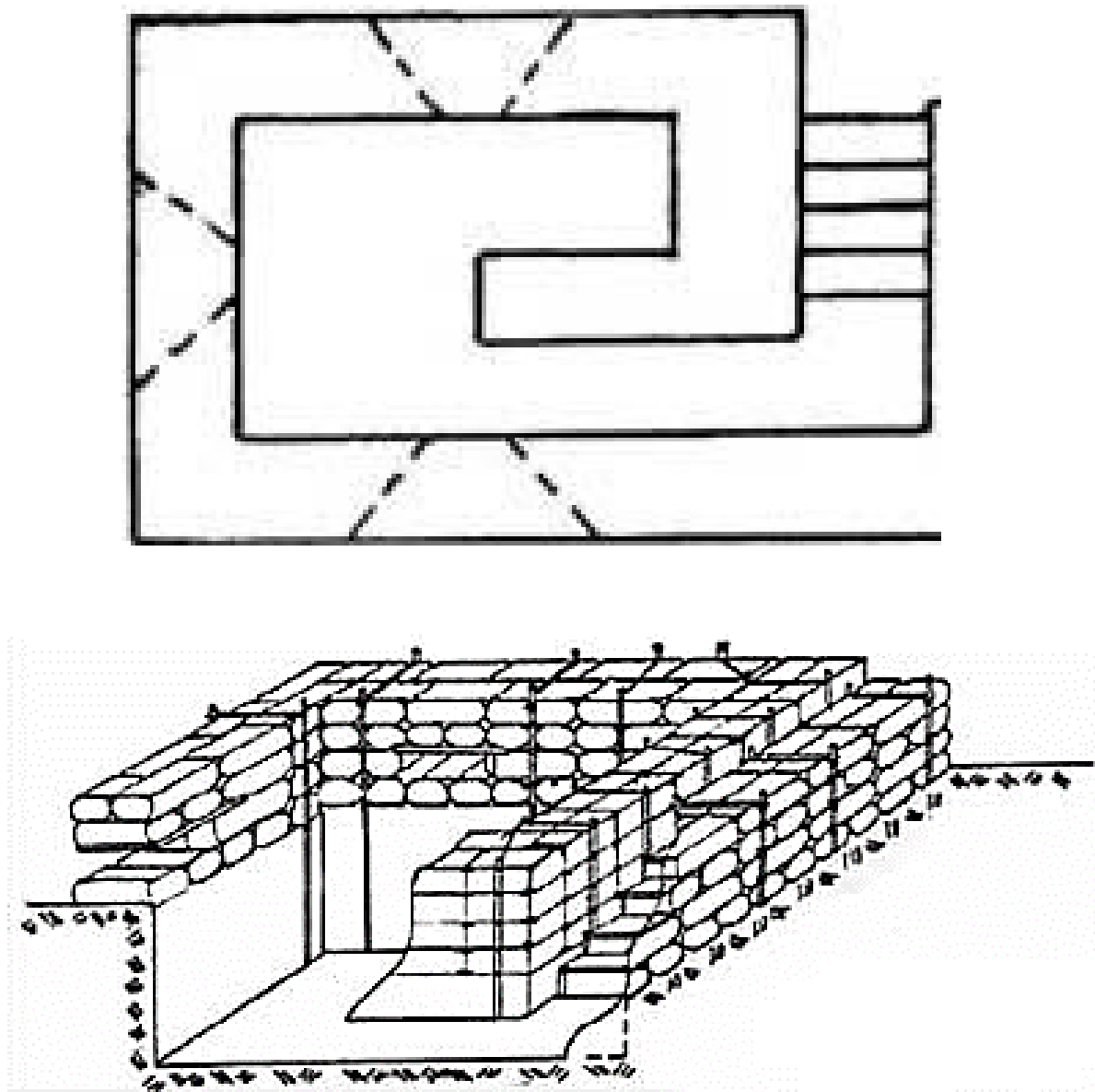
Рис. 70. План будівлі блокпоста
