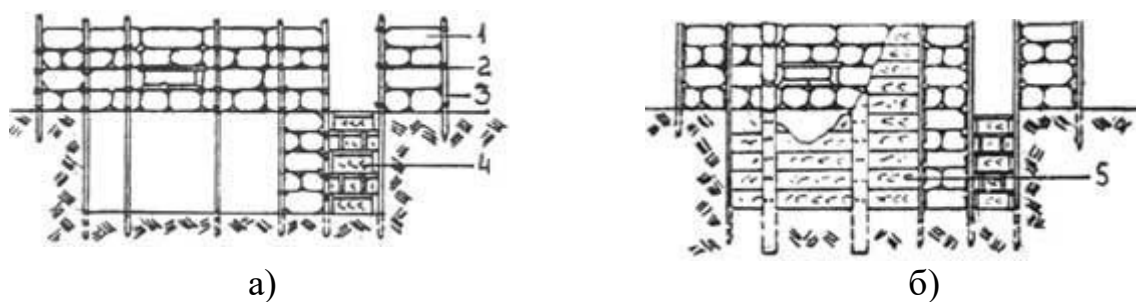
Рис. 69. Будівля блокпоста: а – із МЗ; б – обшитого дошками (1 – МЗ; 2 – дротяна стяжка; 3 – жердини; 4 – східці з дощок; 5 – дошки)
