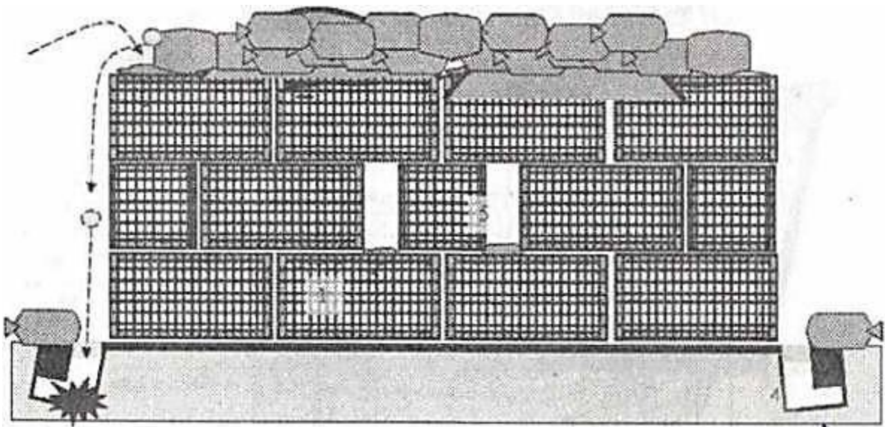
Рис. 71. Блокпост, улаштований із габіонів, покриттям із елементів хвильової сталі та обладнаний протигранатним ровиком (вид спереду).
