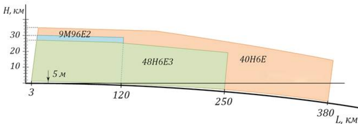
Рис. 1.30. Зони ураження ракет ЗРК С-400
