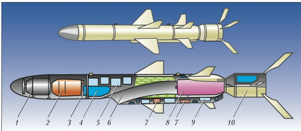
Рис. 3.15. Схема протикорабельної крилатої ракети Х-35:
