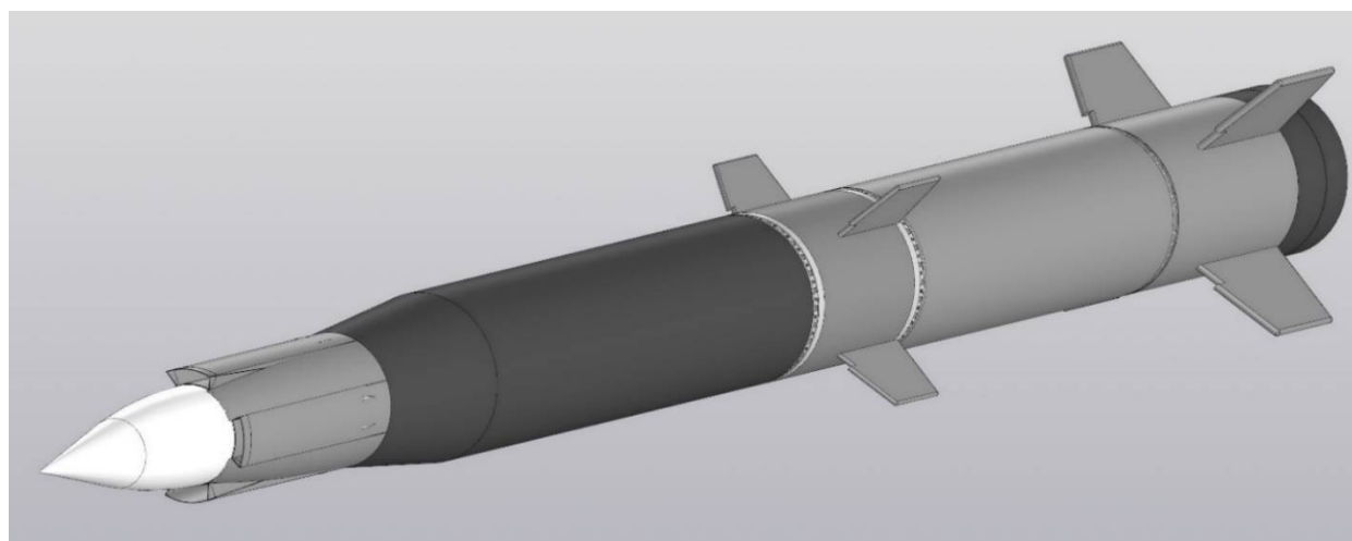
Рис. 3.12. Ракета 3М22 (ймовірно реальна форма) після скидання обтічника
