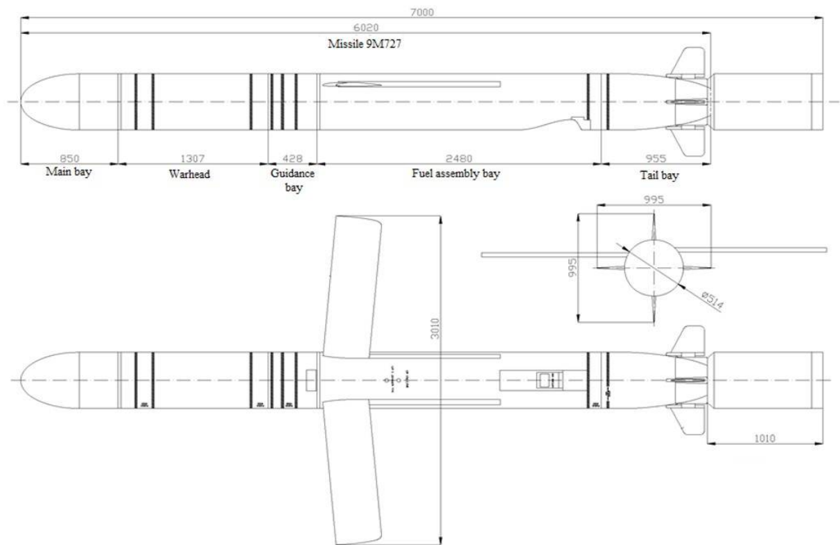
Рис. 3.5. Компонівка крилатої ракети 9М727 (9М728, 9М729)
