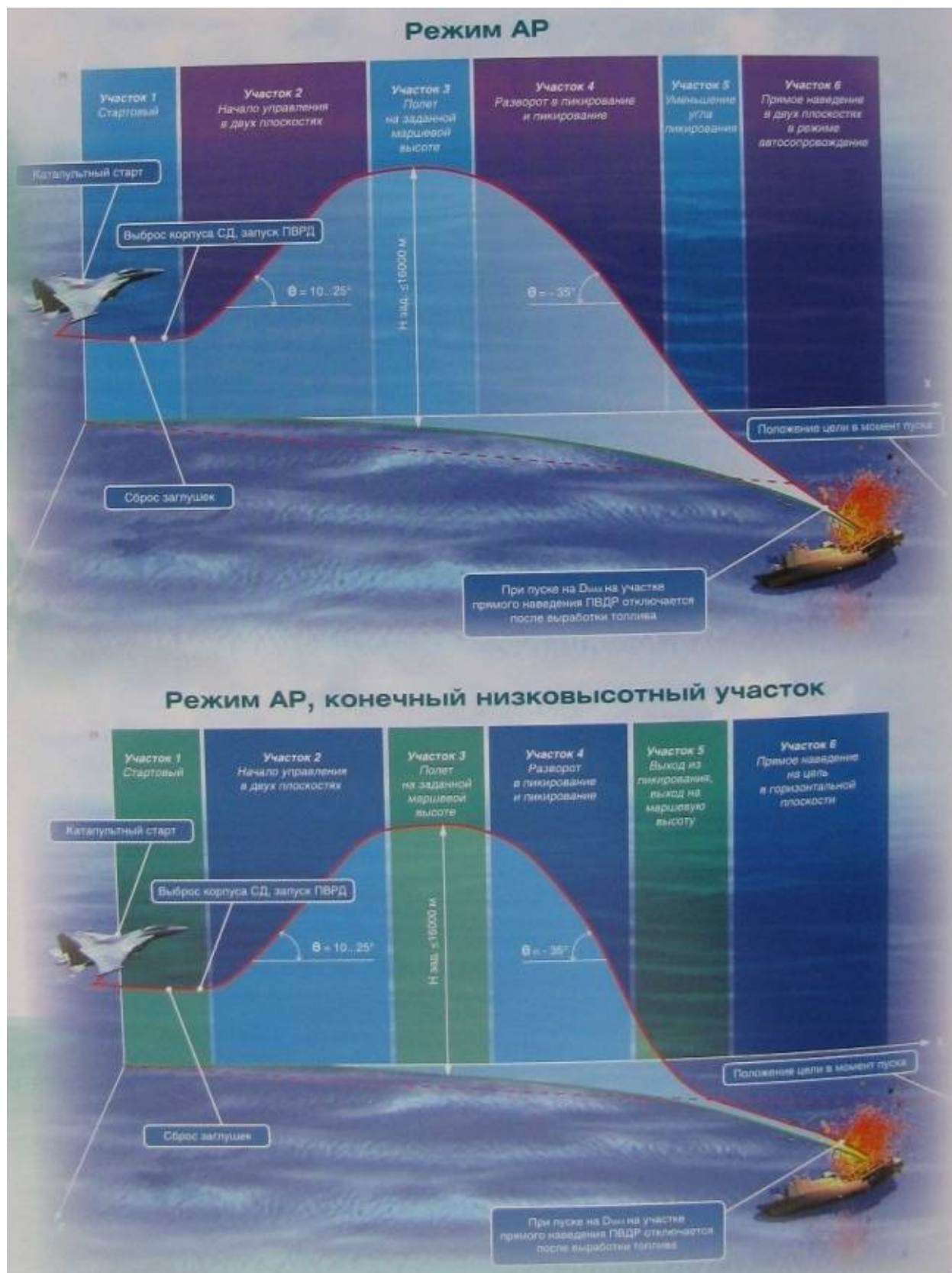
Рис. 2.15. Схема полёту ракеты X-31A
