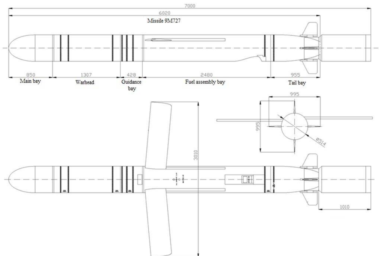
Зображення 4.208. Компоновка ракети 9M727 (9M728) [10]
